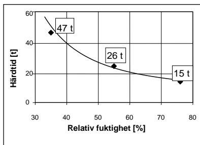
Diagram 1 Härddtid för 500 µm tjock limfilm vid +20°C
