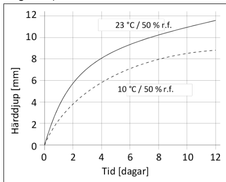
Diagram 1: Härdningshastighet Sikaflex®-221i
