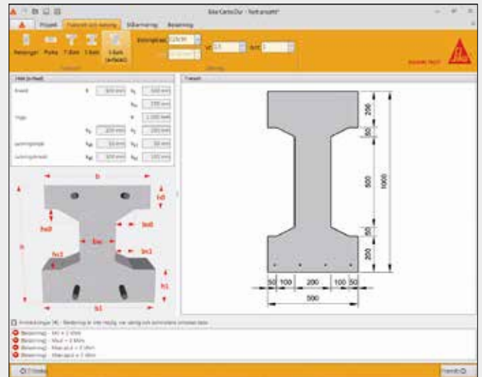
Bestäm hur konstruktionen ser ut.
