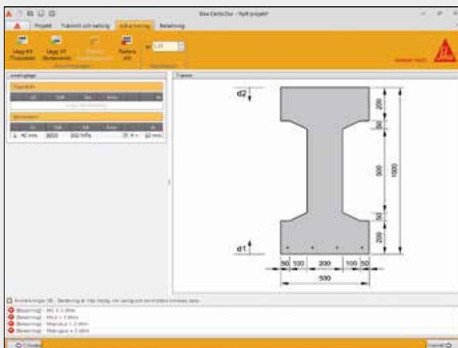
Lägg in hur armeringen ligger.
