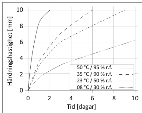
Diagram 1: Härdningshastighet Sikasil® WT-40
