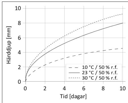
Diagram 1: Härdningshastighet Sikaflex®-591
