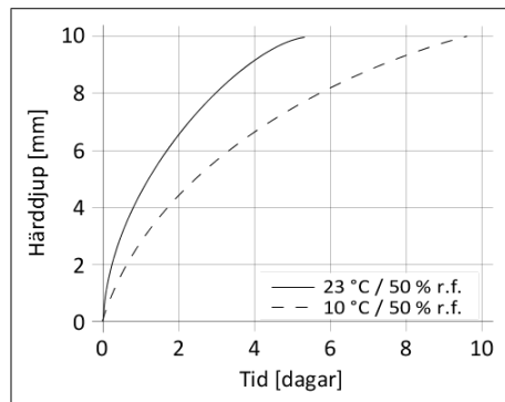
Diagram 1: Härdhastighet Sikaflex®-298 FC
