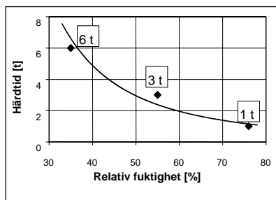
Diagram 1 Härdtid för 500 µm tjock limfilm vid +20°C
