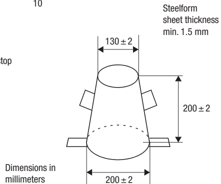
Fig. 5.2.6: Slump cone
