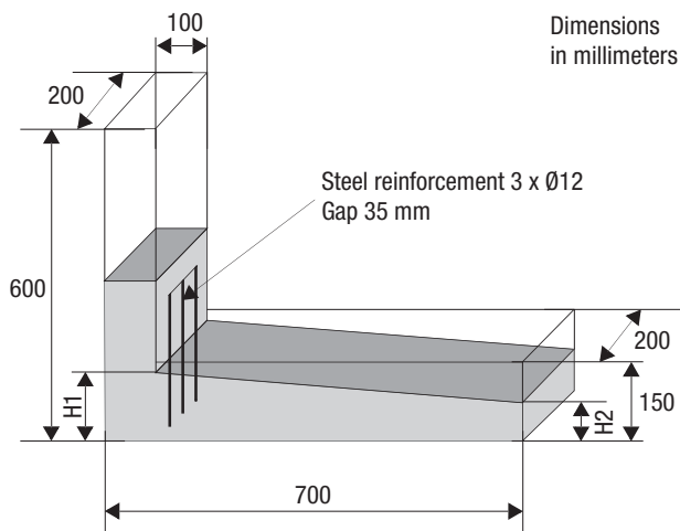
Fig. 5.2.8: L-Box
