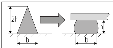
Figur 1: Rekommenderad fogkonfiguration
